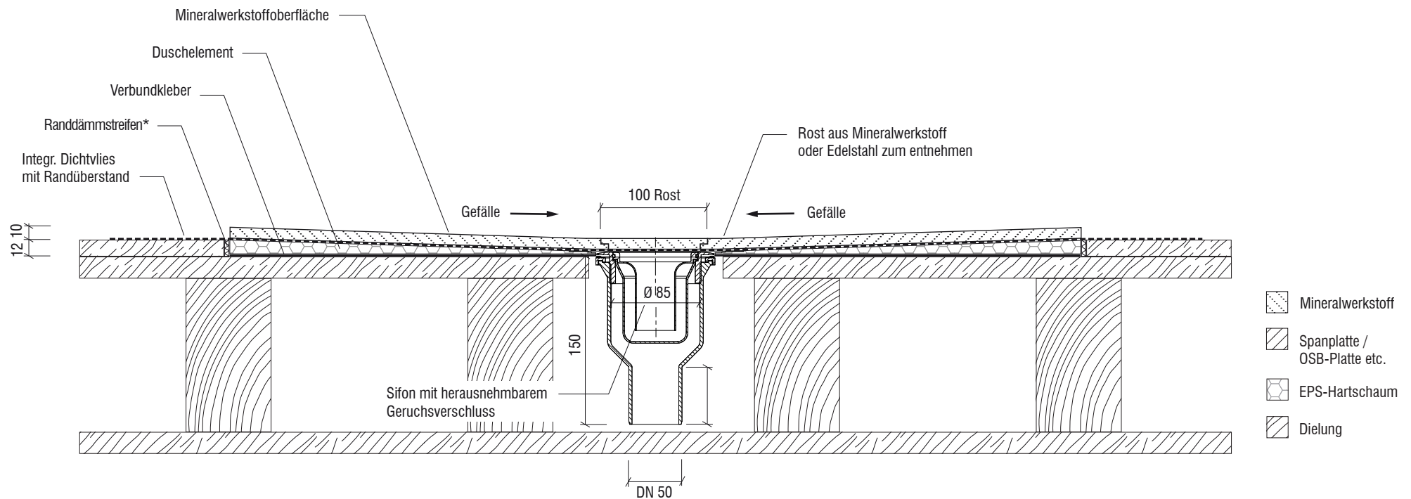
Detail Querschnitt: Maßstab 1:5
