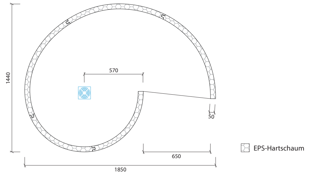
Draufsicht Maßstab 1:20
