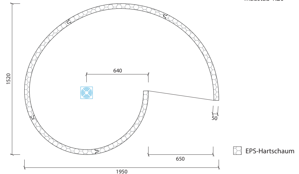
Draufsicht Maßstab 1:20
