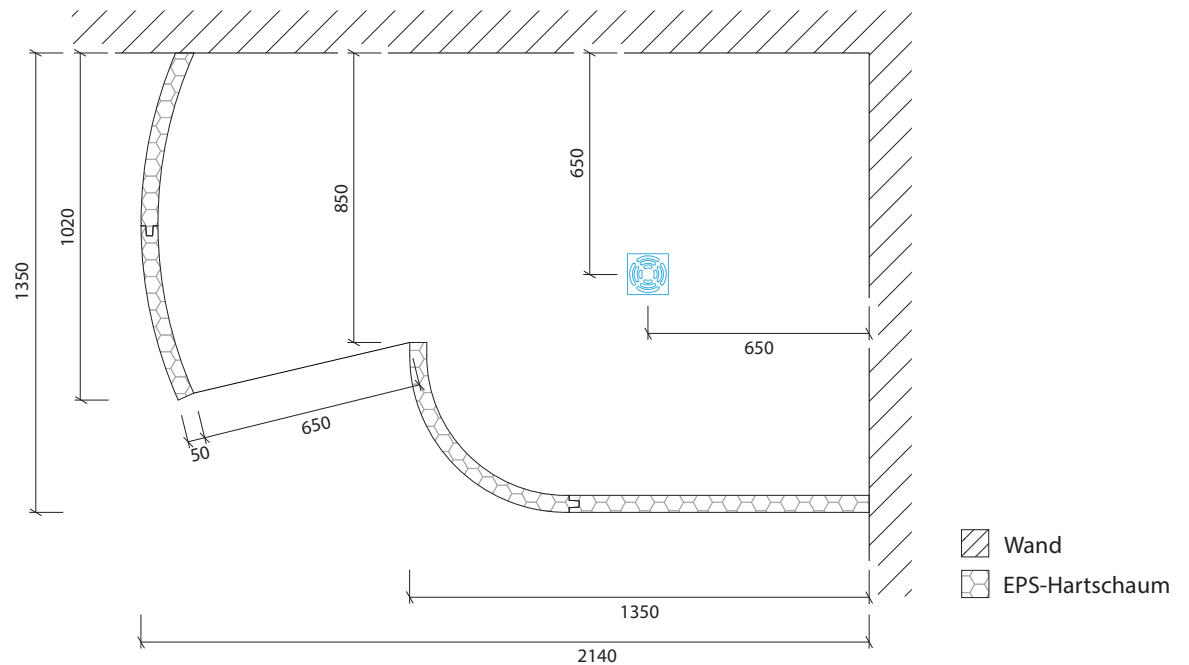
Draufsicht Maßstab 1:20
